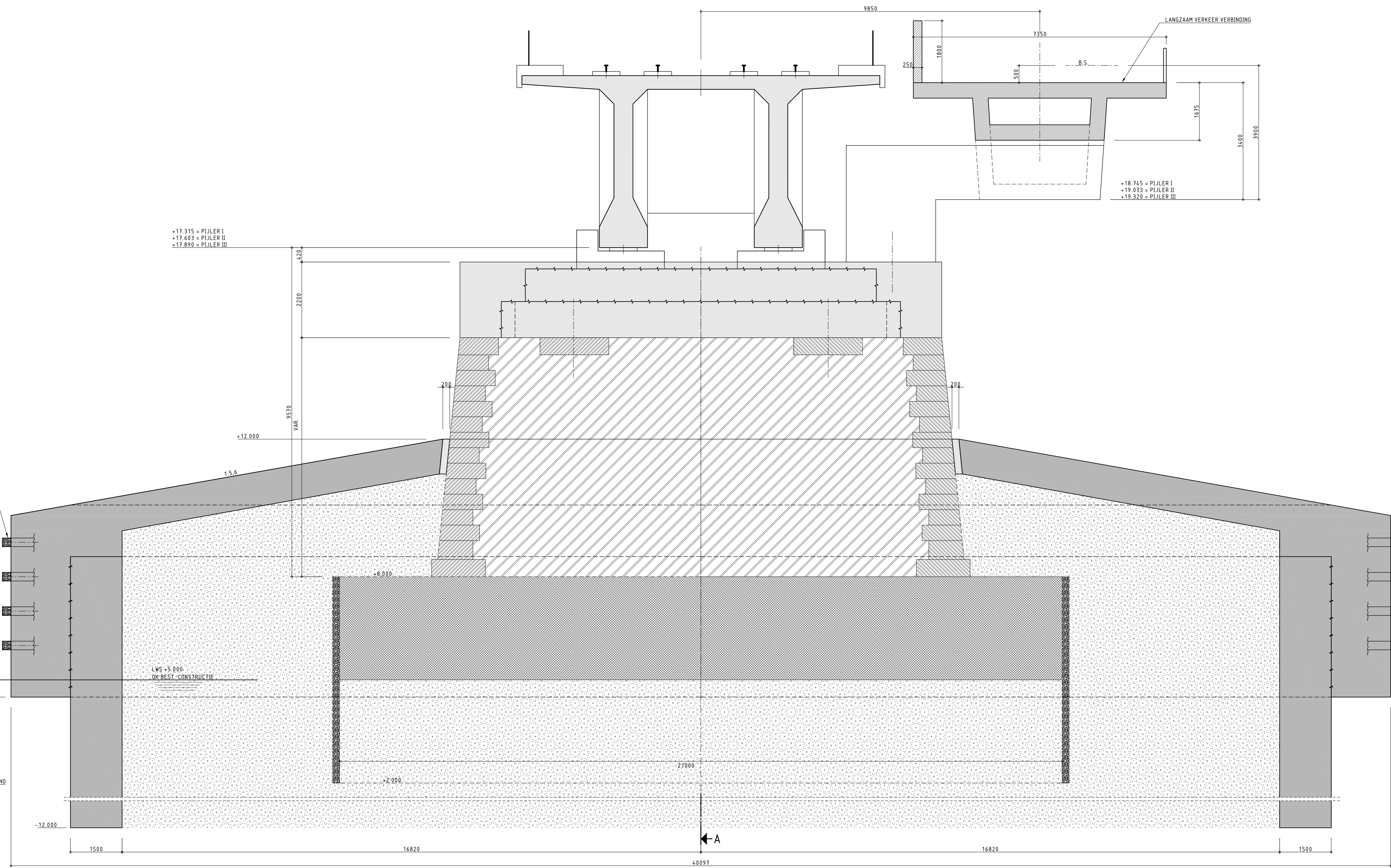
LANGSDOORSNEDE NIEUWE SITUATIE SCHAAL 1:100
