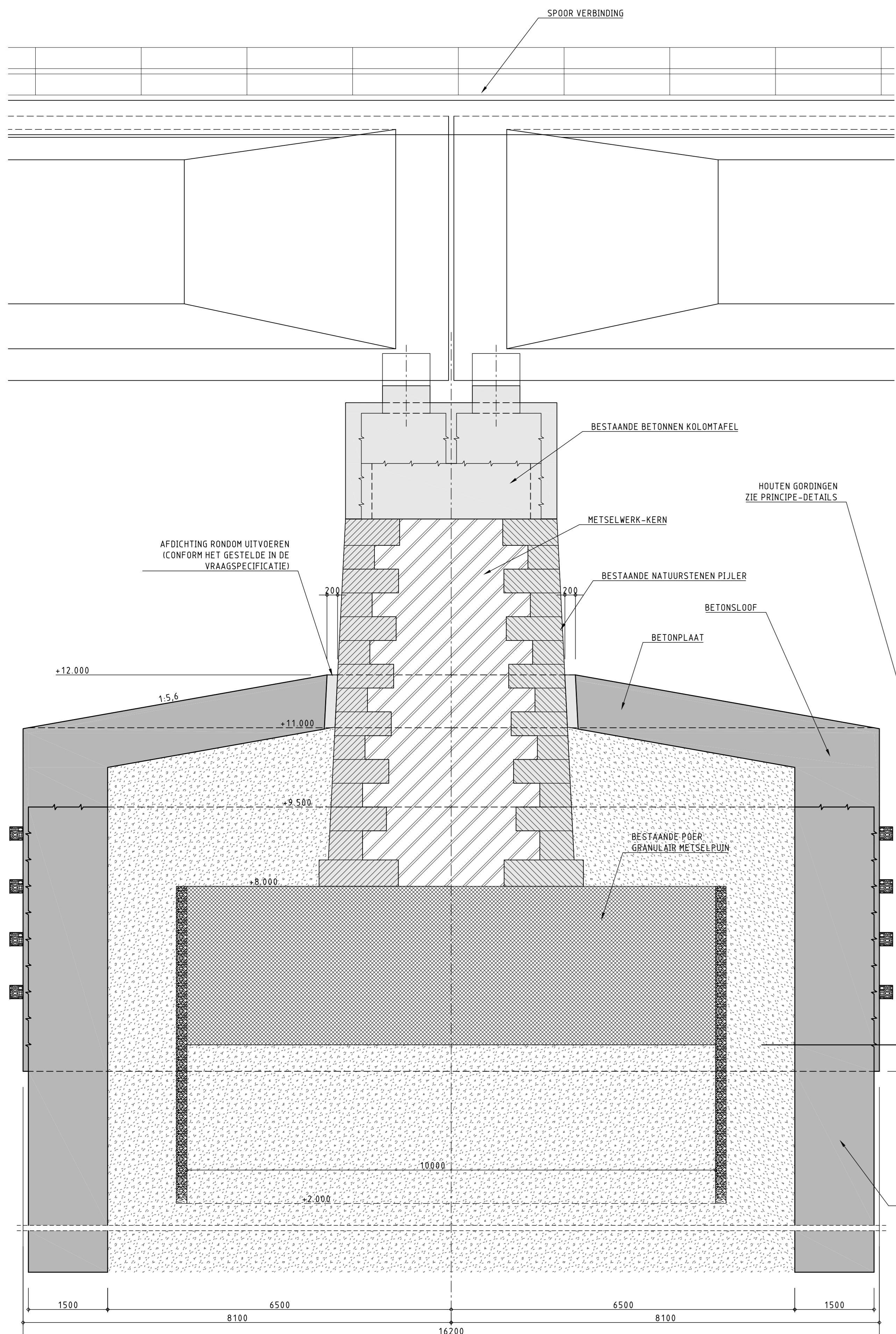
DWARSDOORSNEDE NIEUWE SITUATIE SCHAAL 1:50
